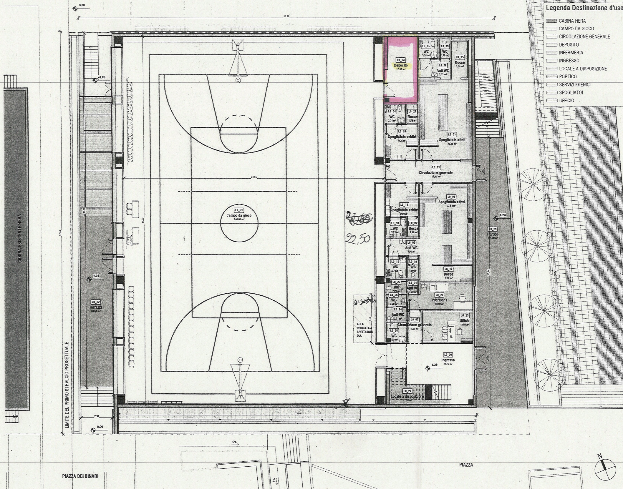
PIANTA PIANO TERRA - LAYOUT COMPETIZIONE scala - 1:100
