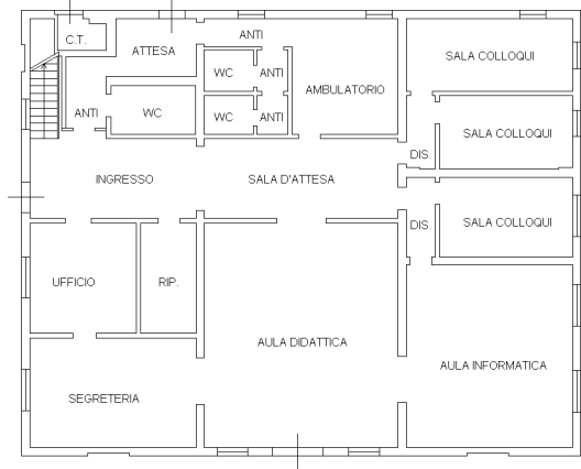
PIANO TERRA H = 4,35 m.
