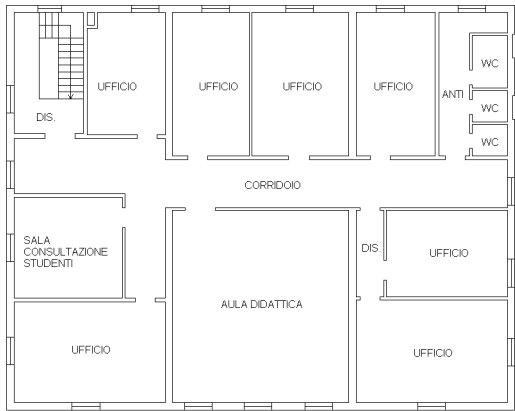
PIANO PRIMO H = 2,75 m.
